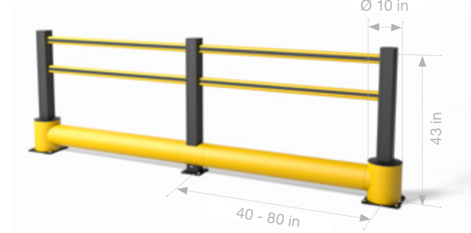
TB 260 PLUS 21.20 kJ
