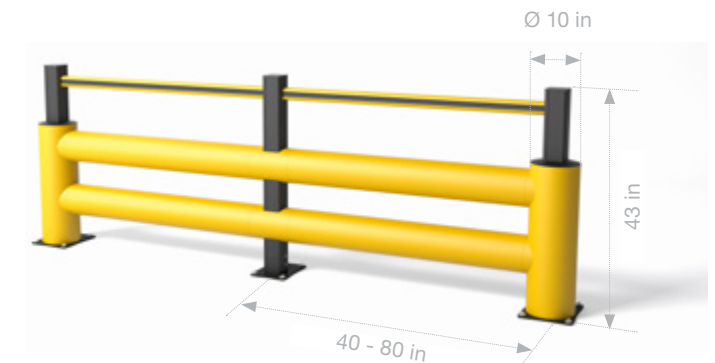
TB 400 DOUBLE PLUS 39.10 kJ
